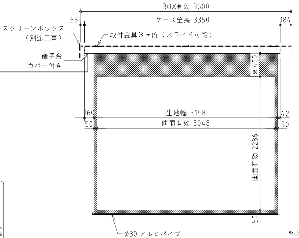
外観図 S=1/40
