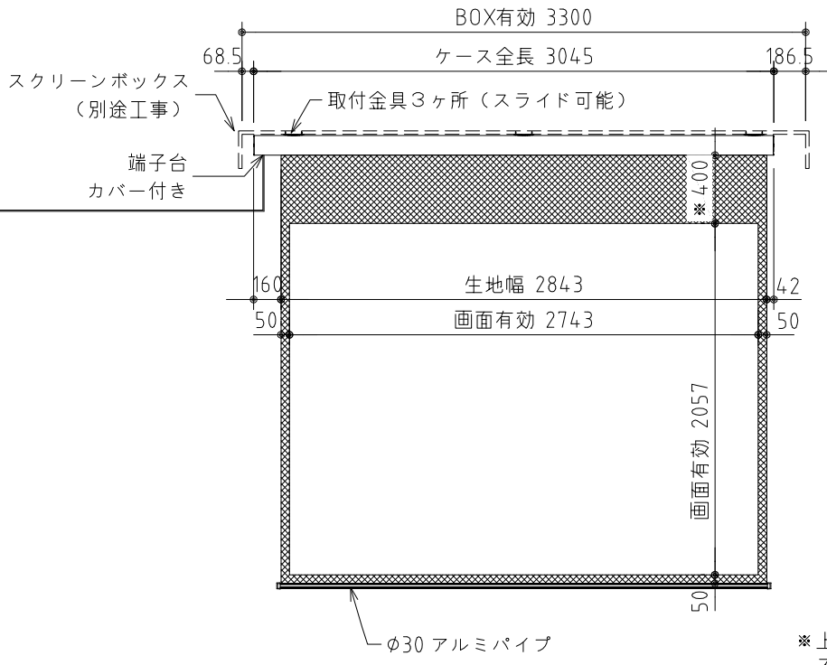
外觀図 S=1/40
