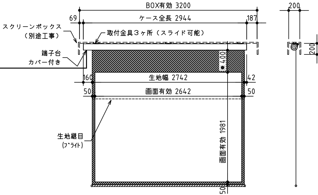
外観図 S=1/40
