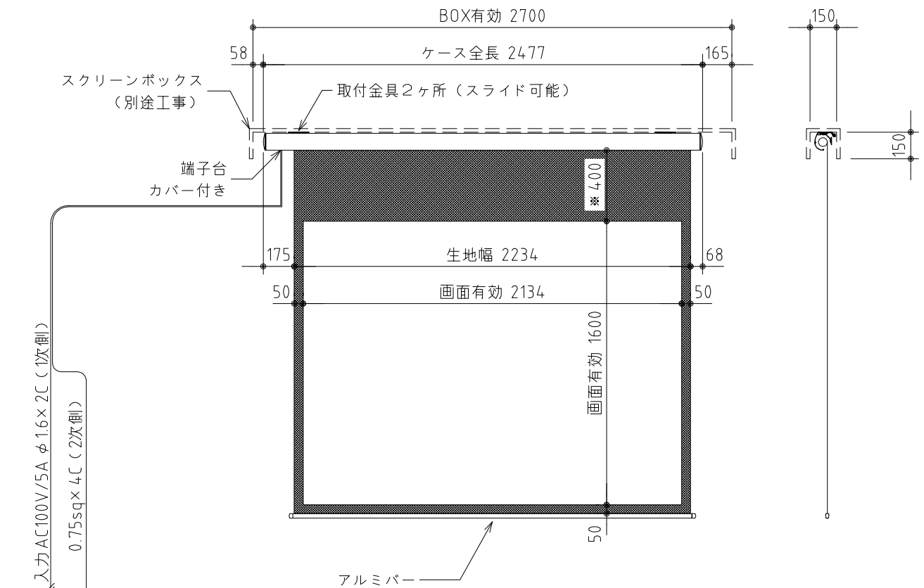
外観図 S=1/30
