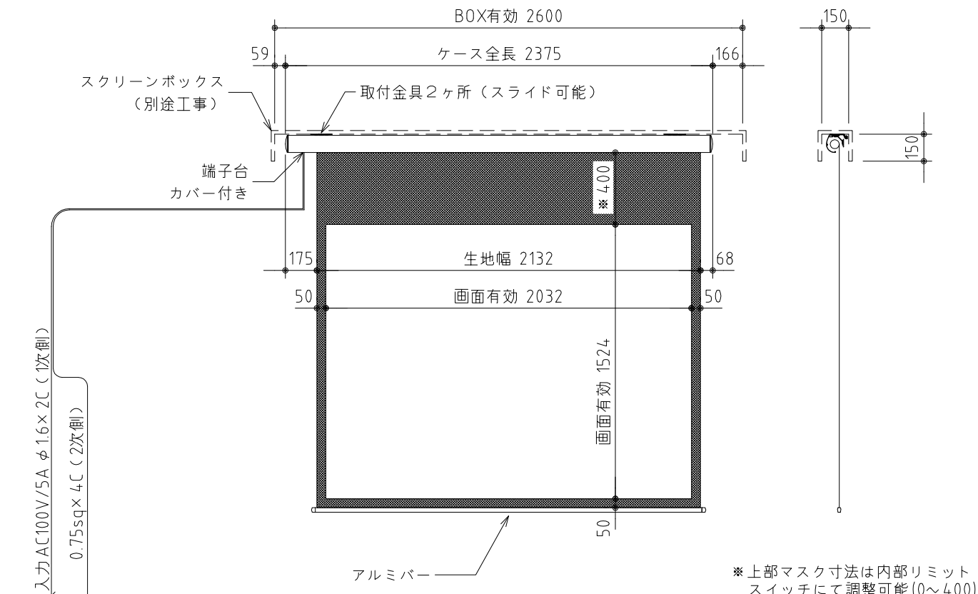
外観図 S=1/30
