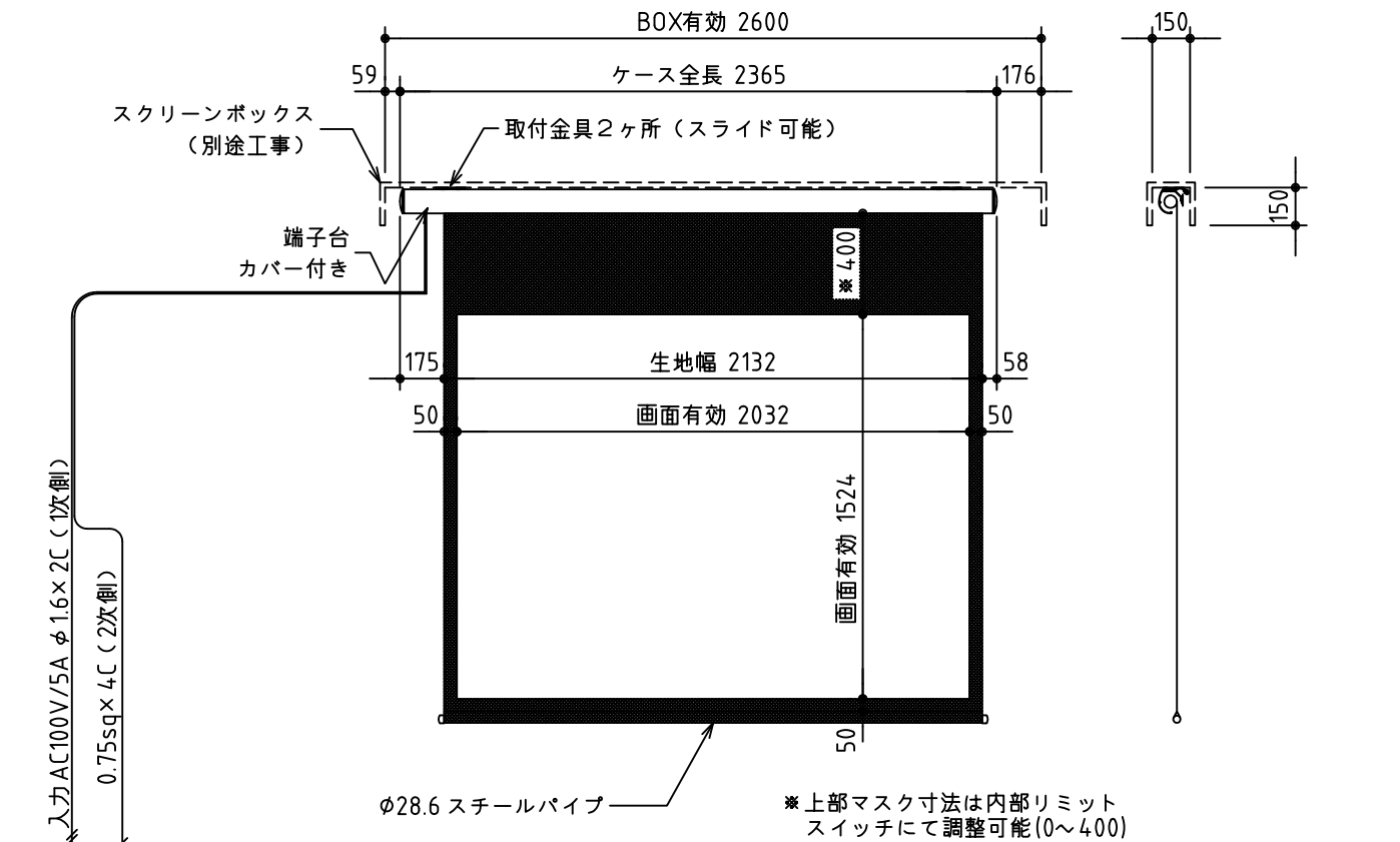
外観図 S=1/30
