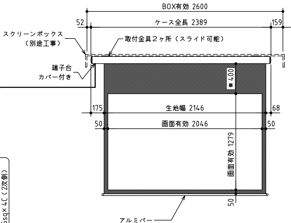
外観図 S=1/30
