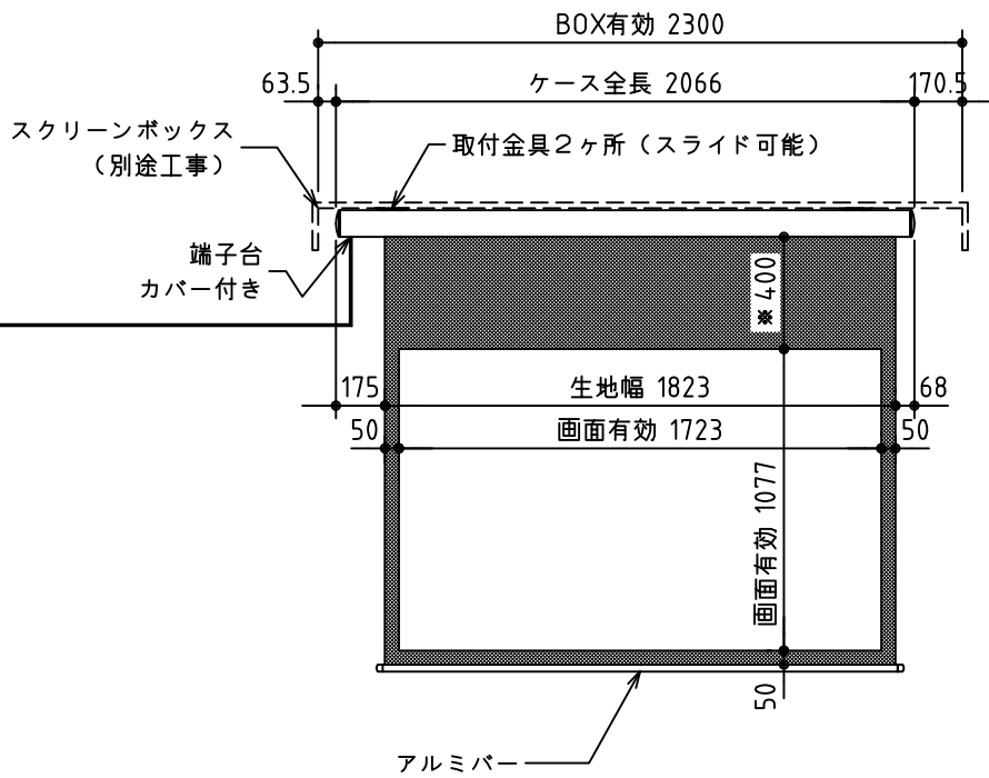
外観図 S=1/30
