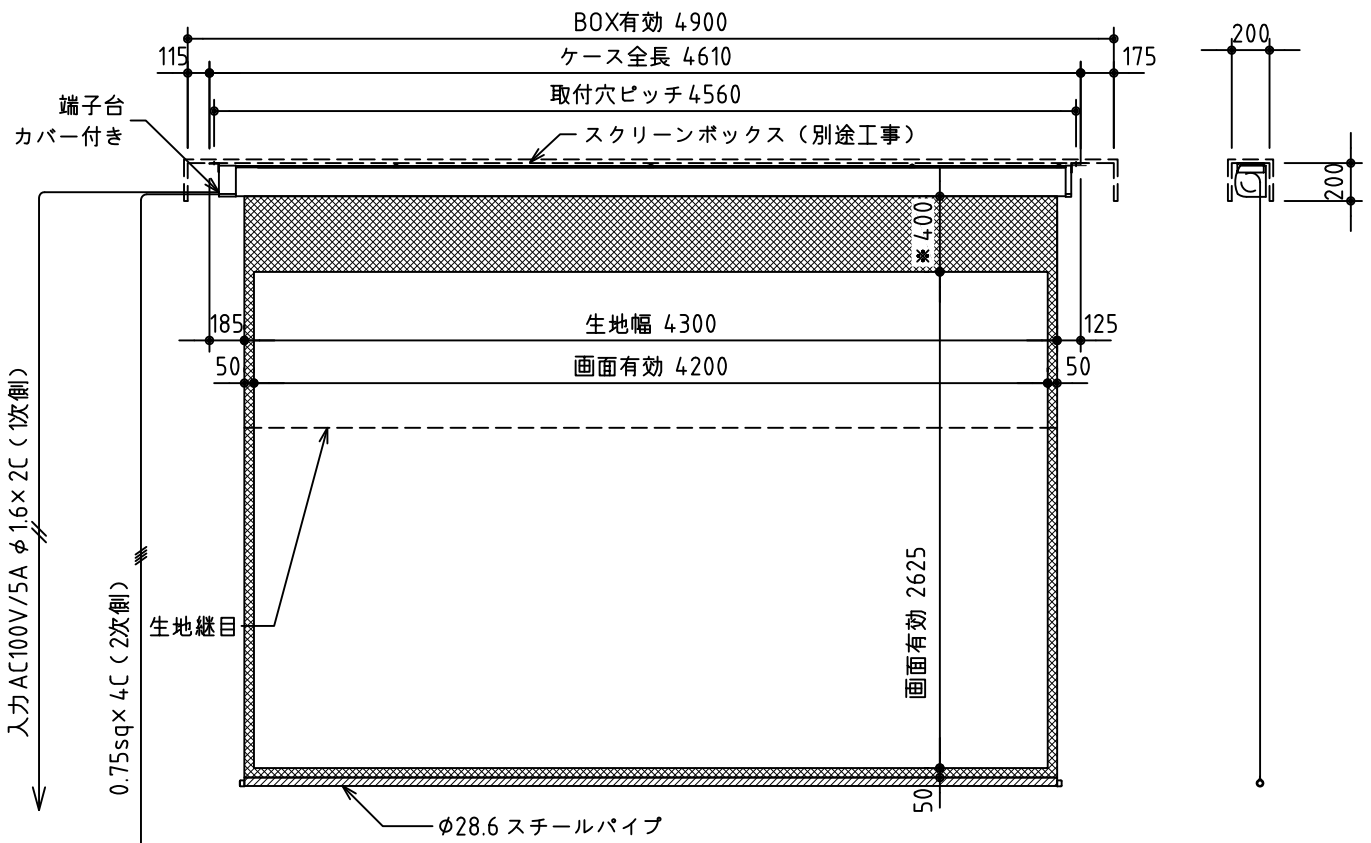
外観図 S=1/40
