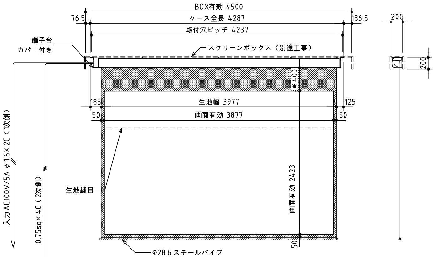
外観図 S=1/40
