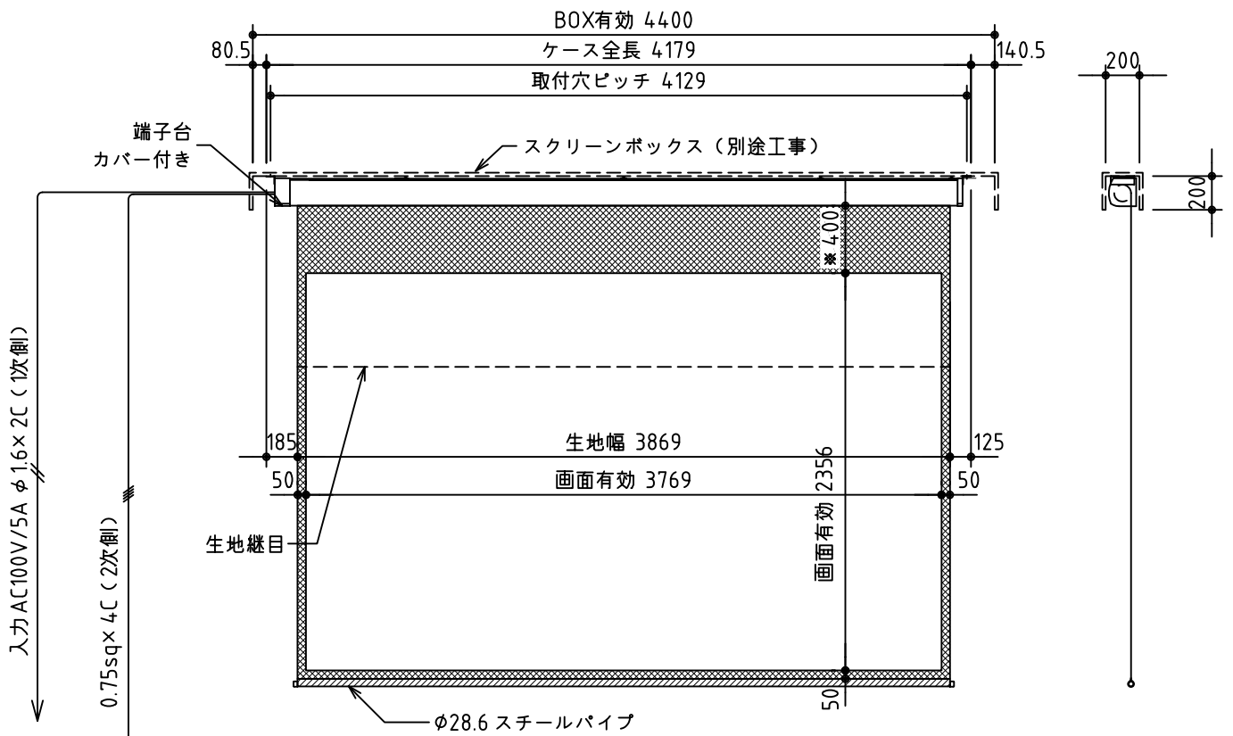
外觀図 S=1/40
