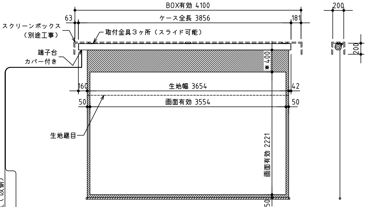
外観図 S=1/40
