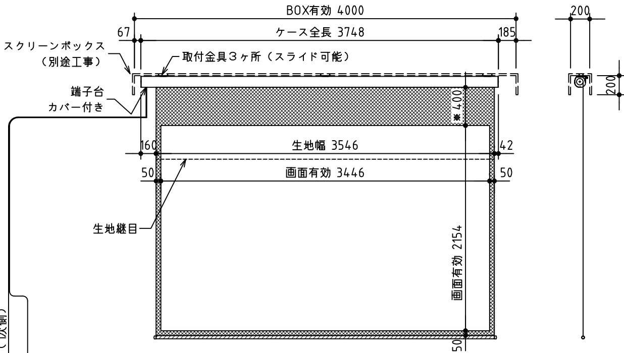
外観図 S=1/40
