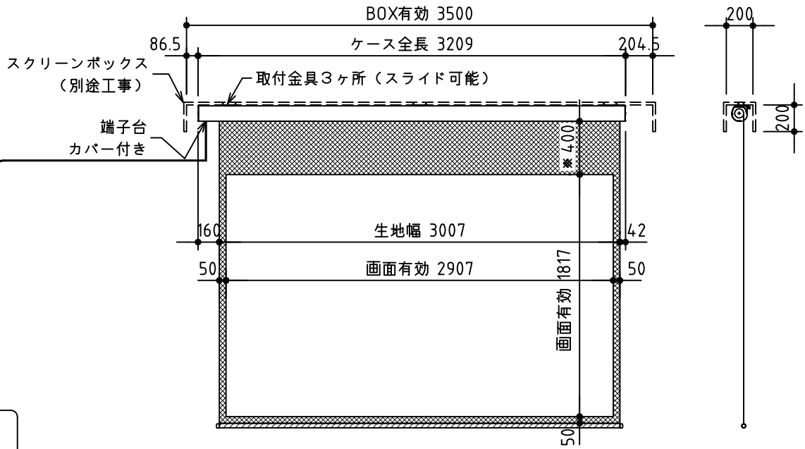
外觀図 S=1/40
