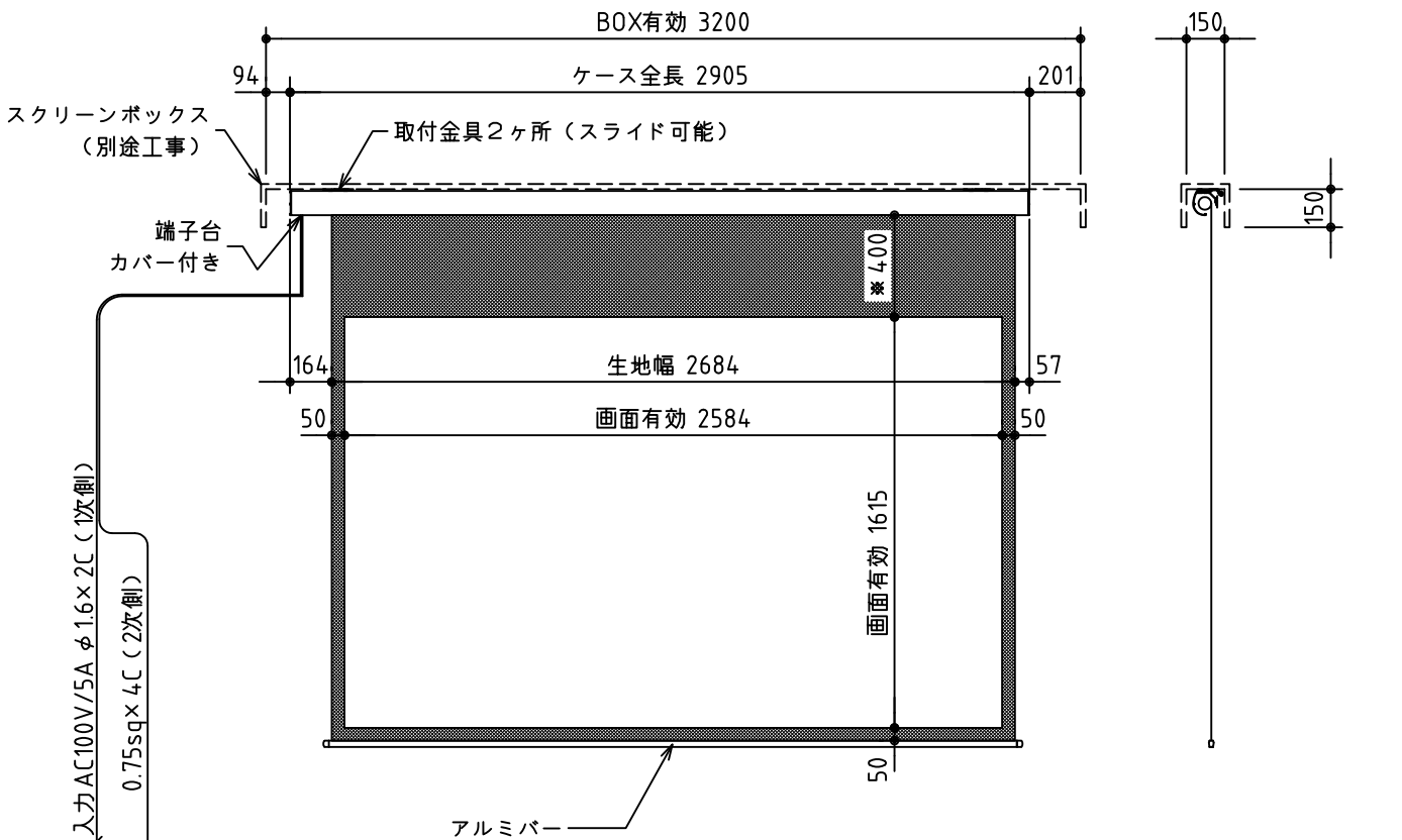
外観図 S=1/30
