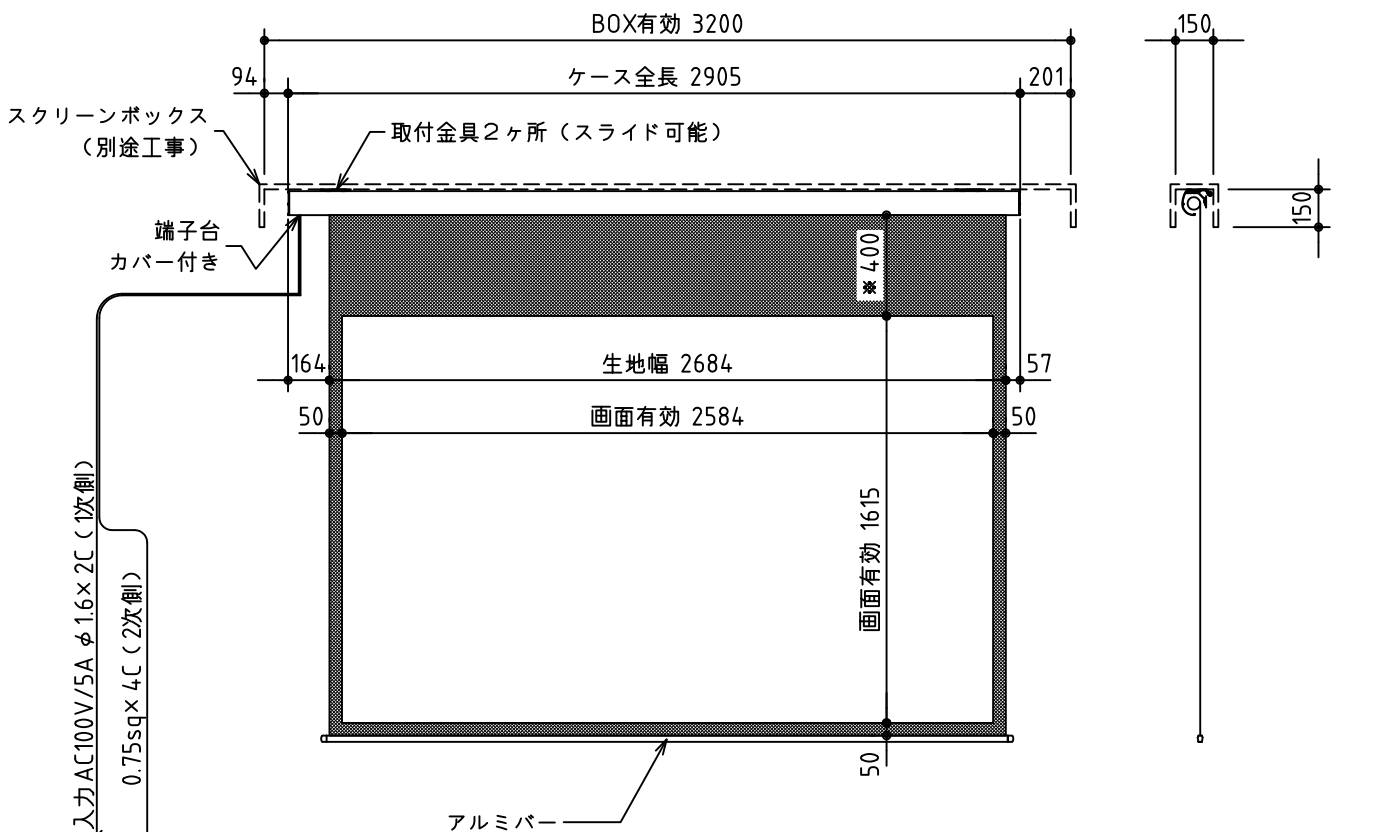
外観図 S=1/30
