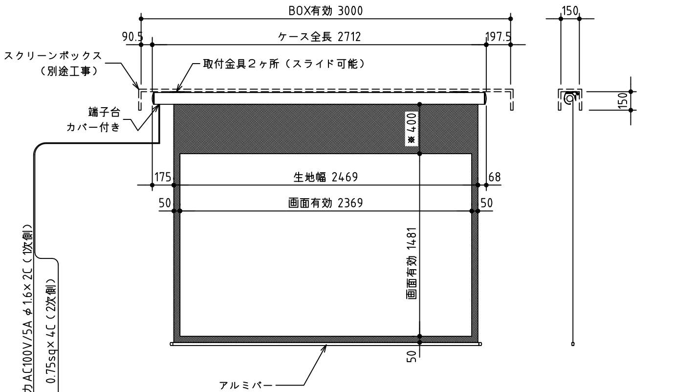
外観図 S=1/30
