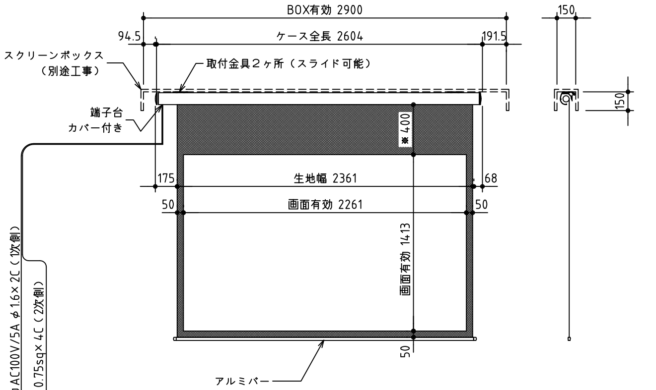
外觀図 S=1/30
