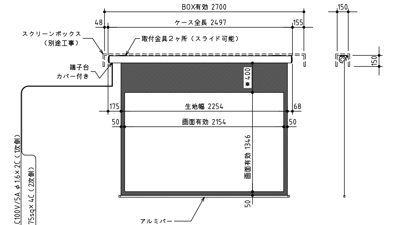
外観図 S=1/30
