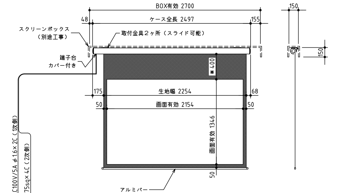
外観図 S=1/30
