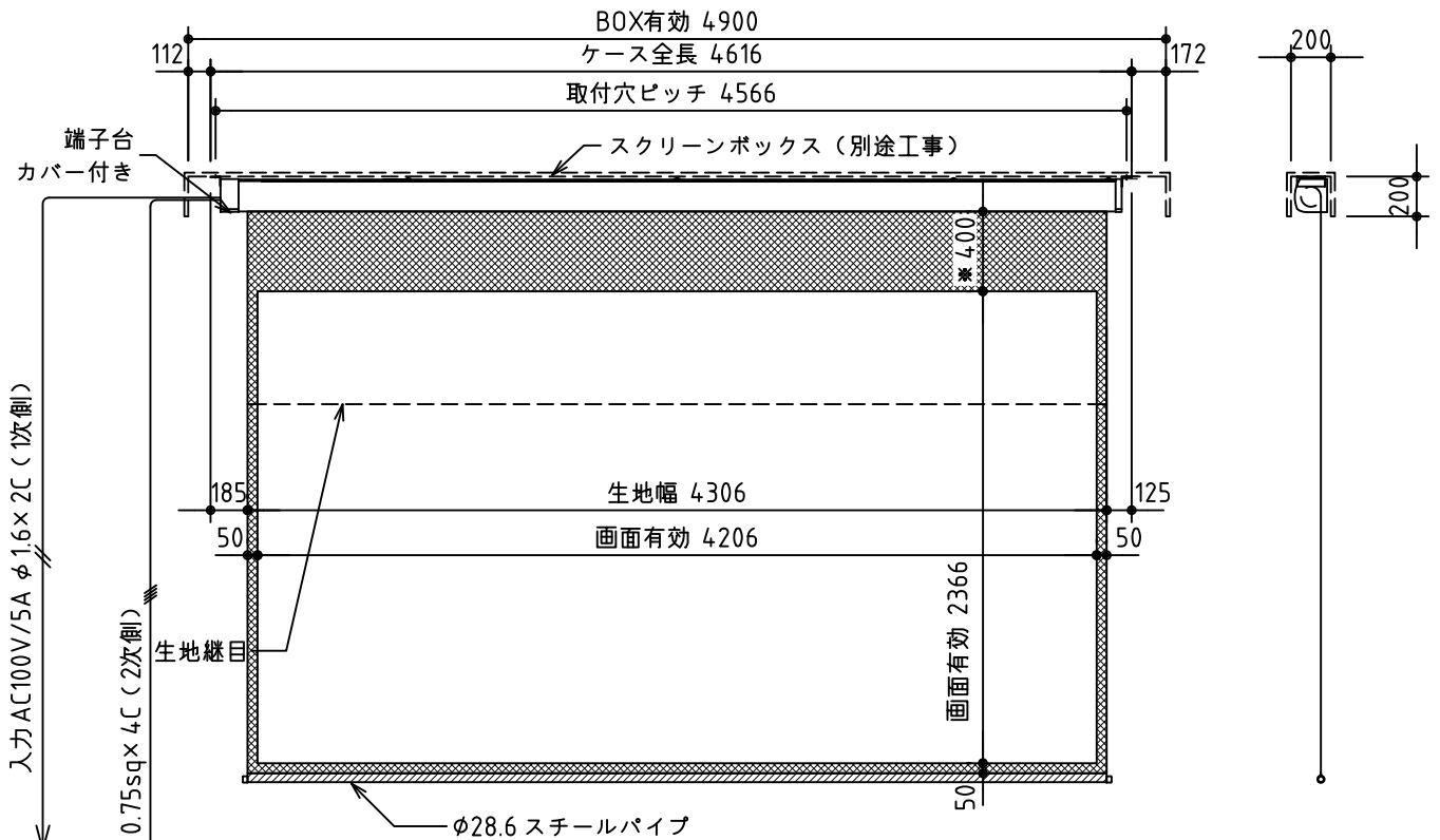
外觀図 S=1/40
