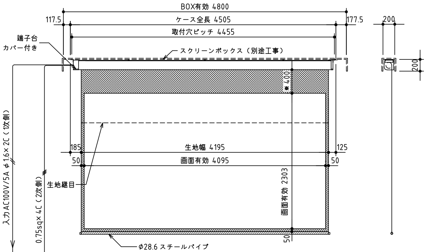
外觀図 S=1/40
