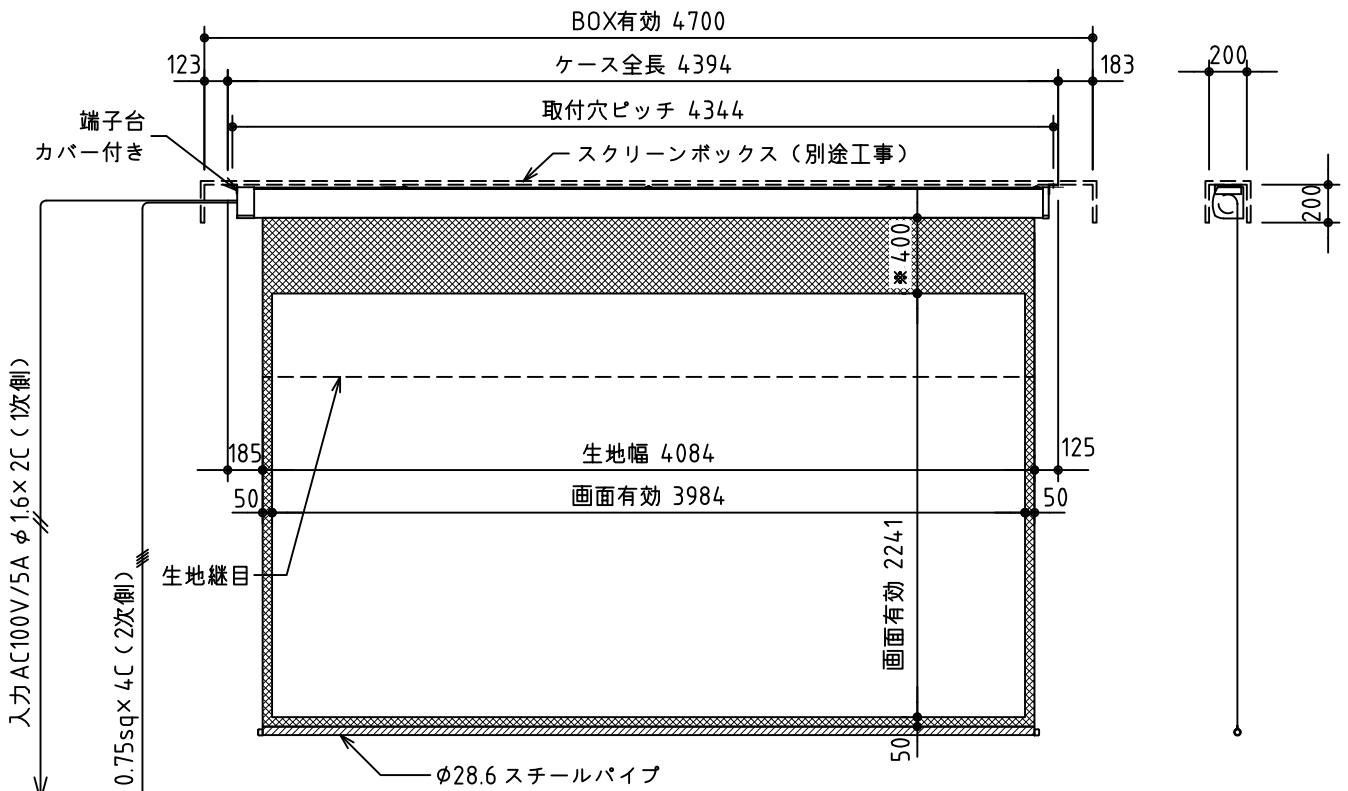
外観図 S=1/40
