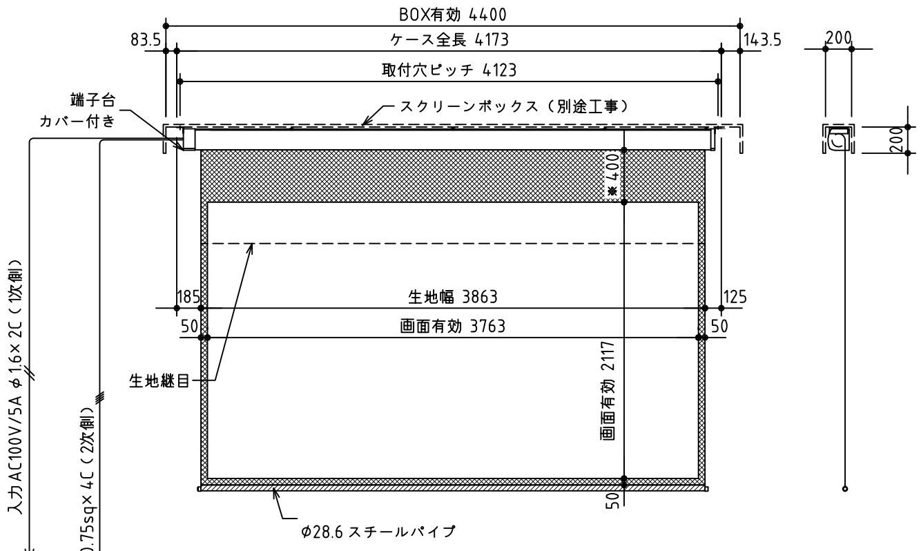
外観図 S=1/40
