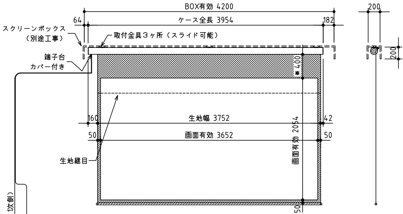
外觀図 S=1/40
