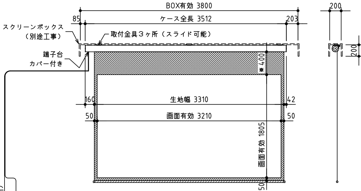
外觀図 S=1/40
