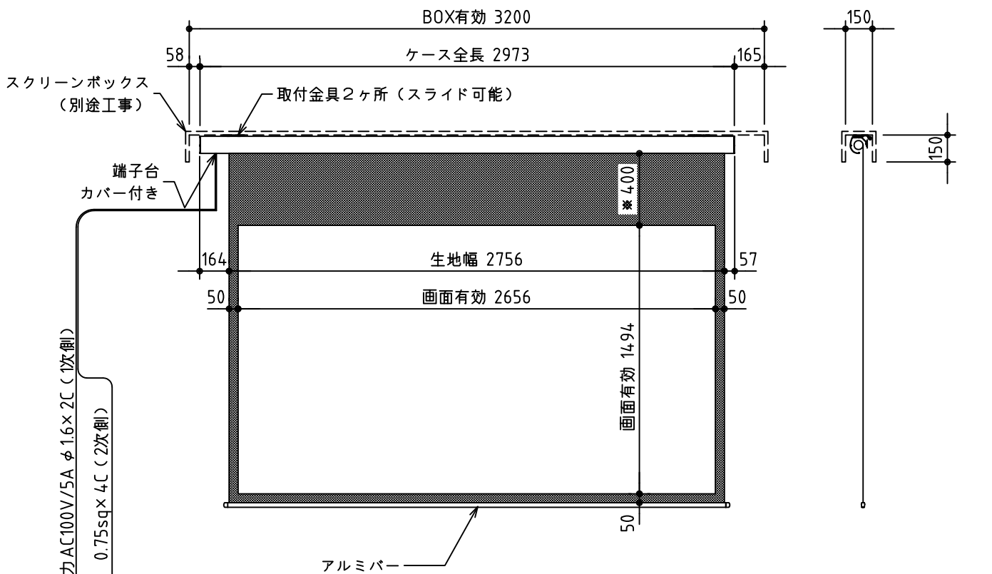
外觀図 S=1/30
