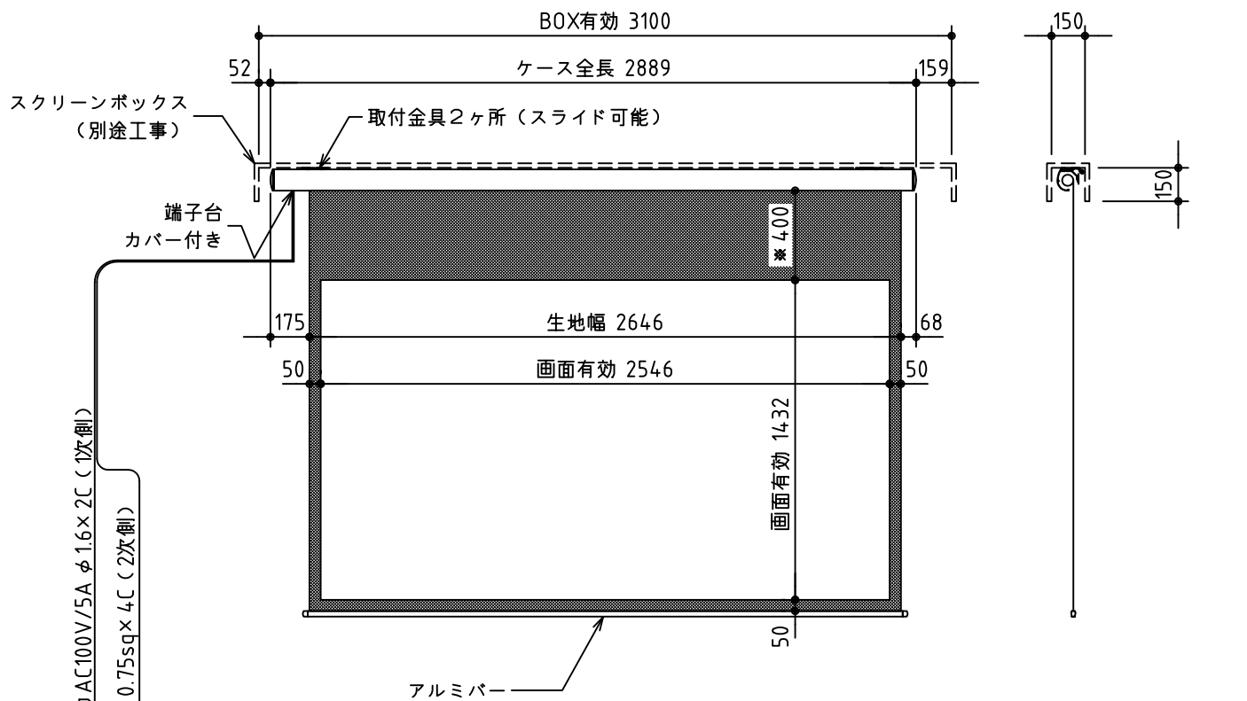
外観図 S=1/30
