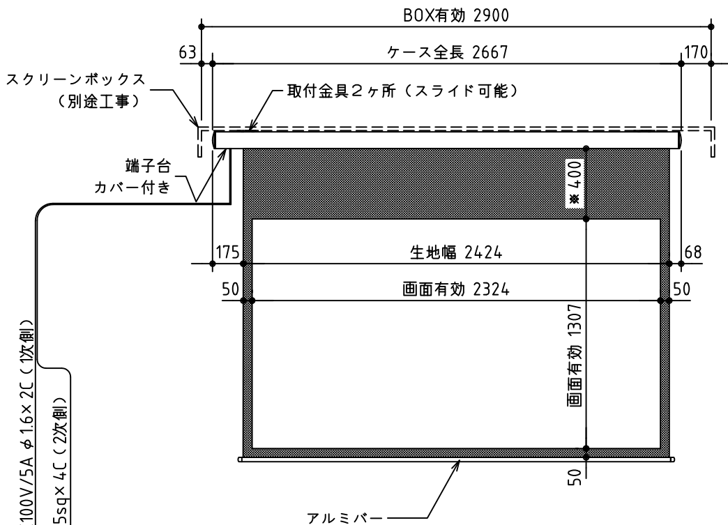
外観図 S=1/30
