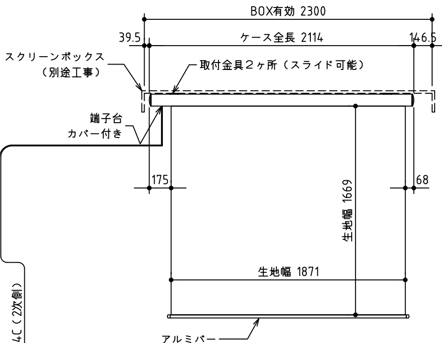
外観図 S=1/30
