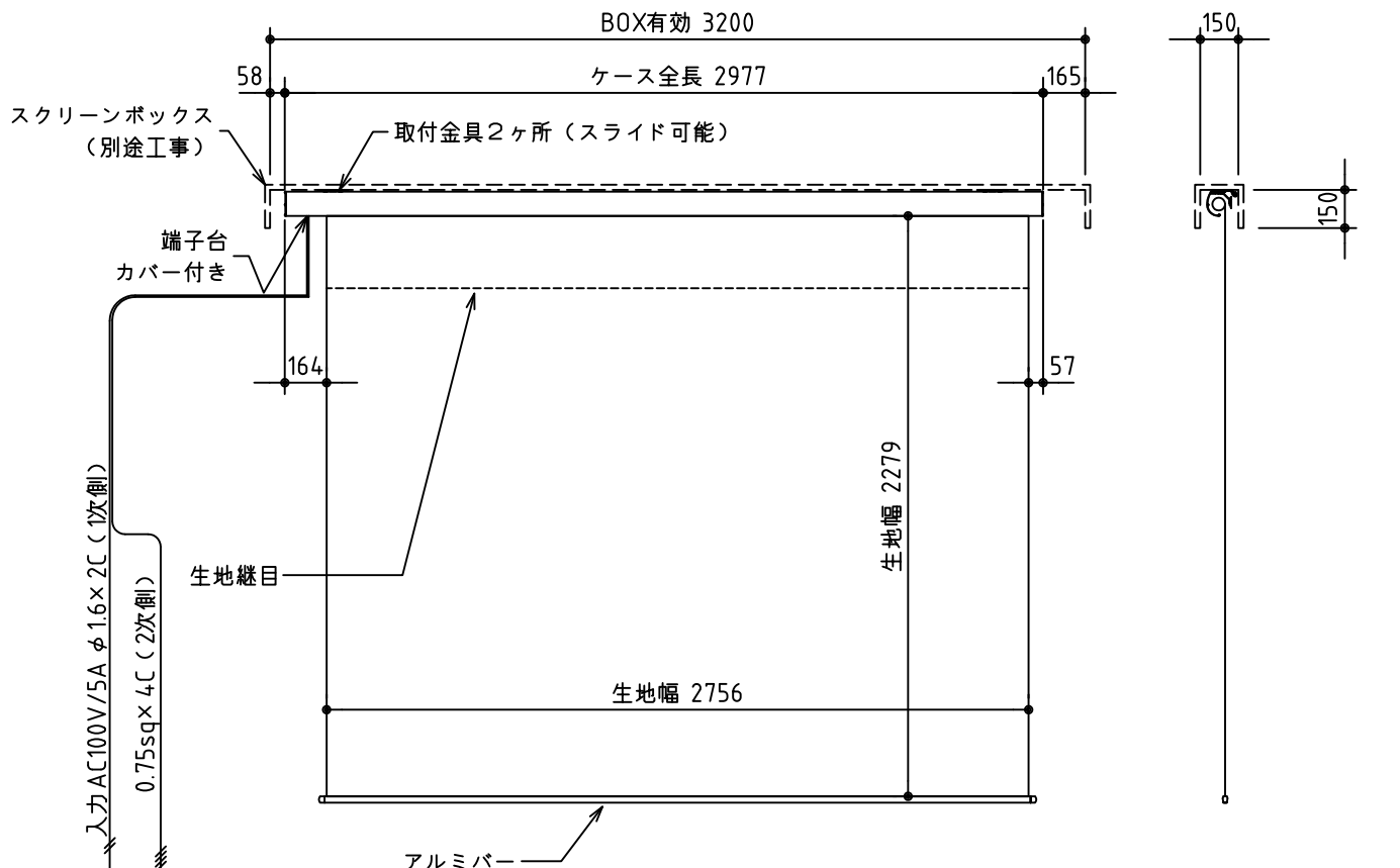
外観図 S=1/30
