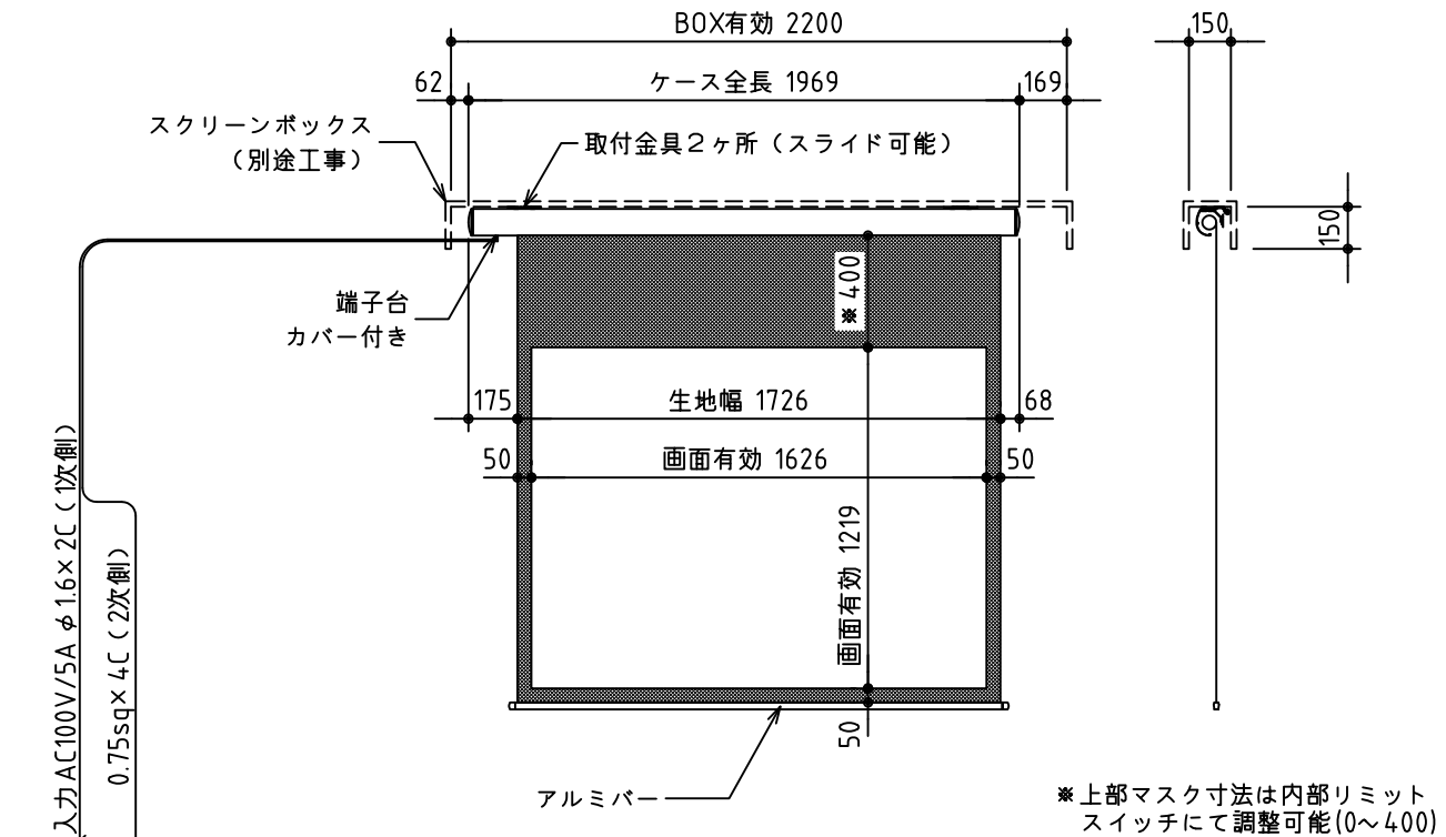
外観図 S=1/30
