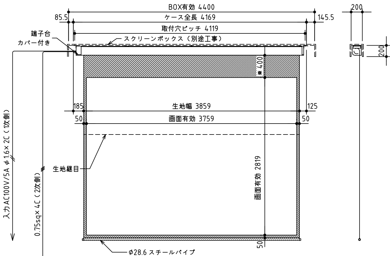
外觀図 S=1/40
