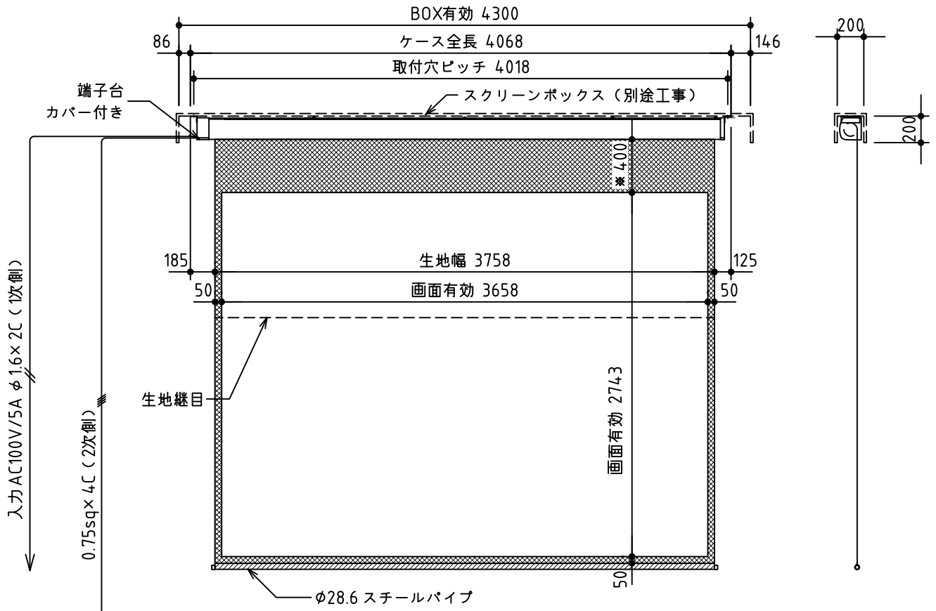
外観図 S=1/40
