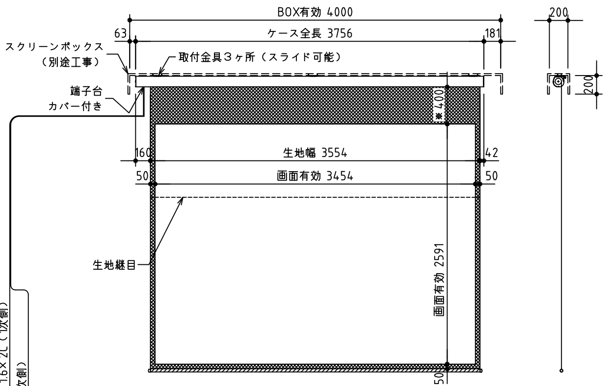
外観図 S=1/40
