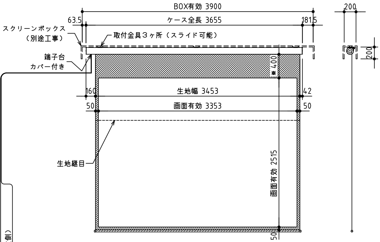
外観図 S=1/40
