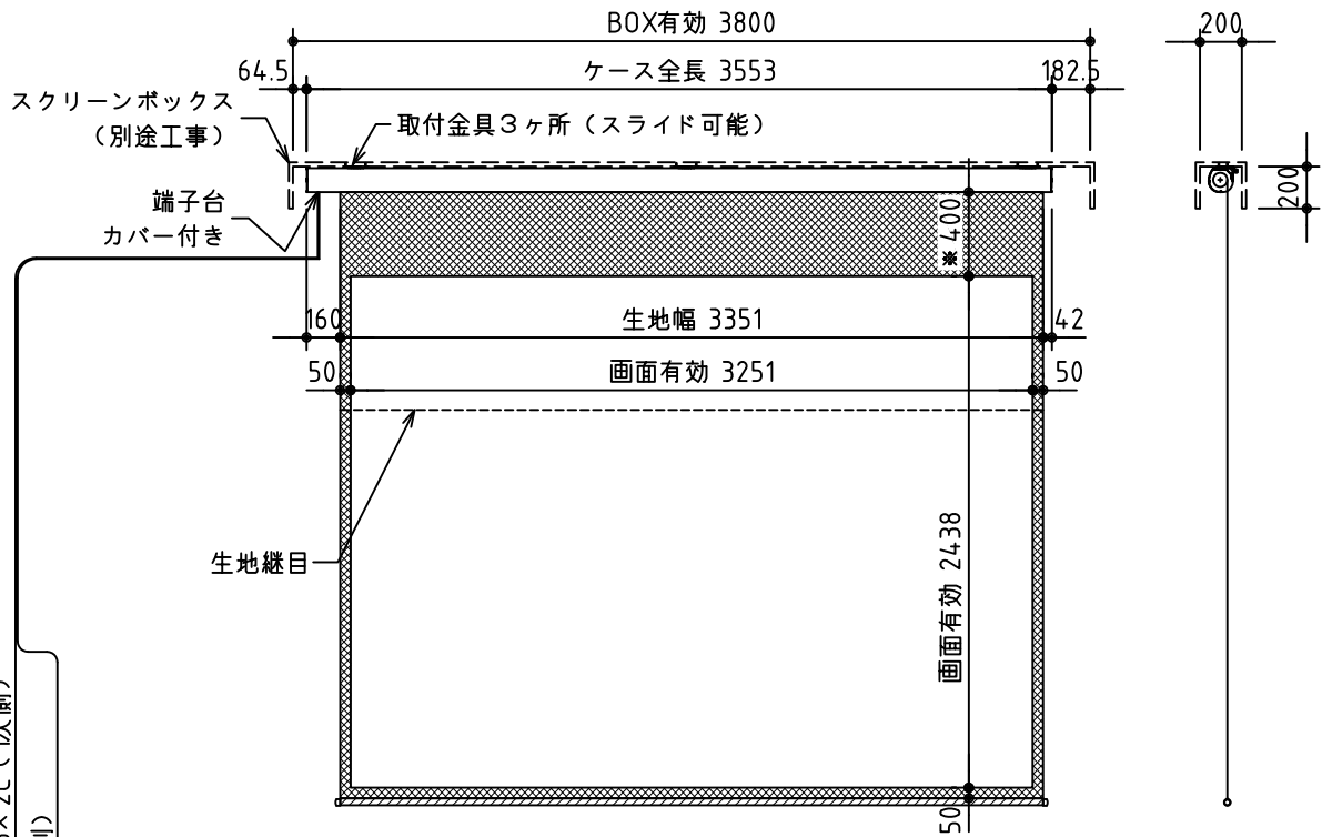
外観図 S=1/40
