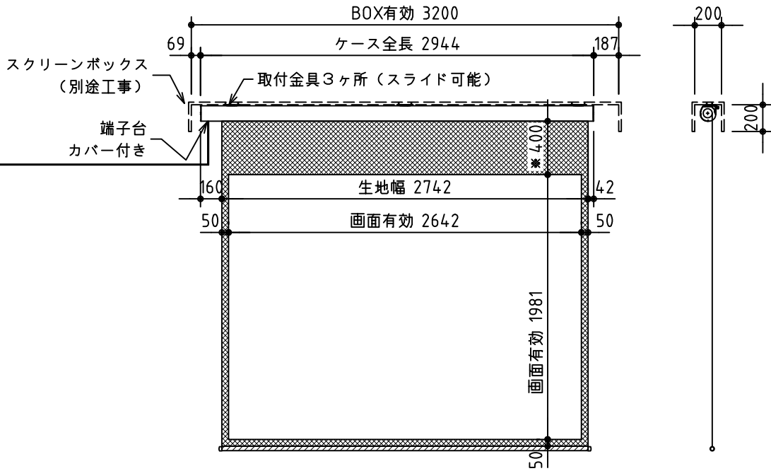
外観図 S=1/40
