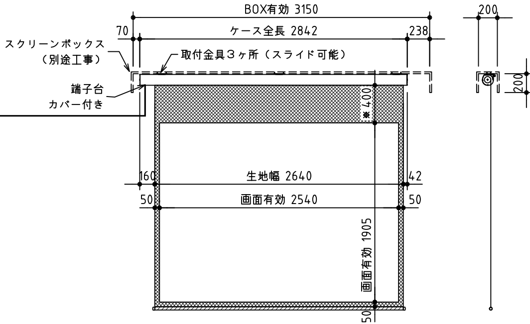
外観図 S=1/40
