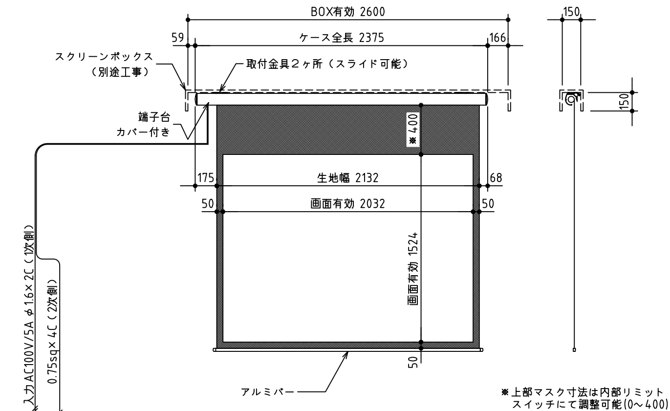
外観図 S=1/30
