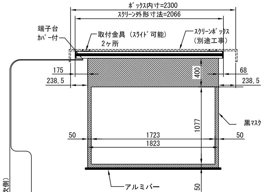
外観図 1/30
