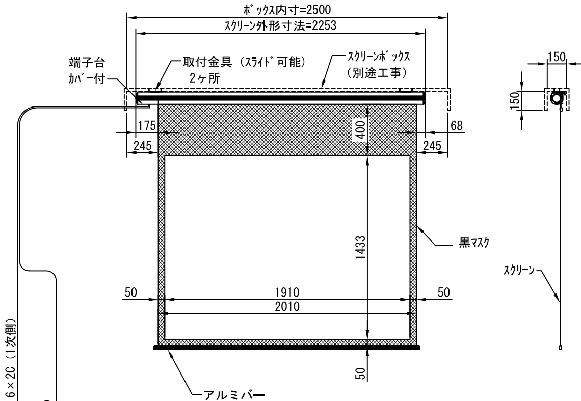
外觀図 1/30
