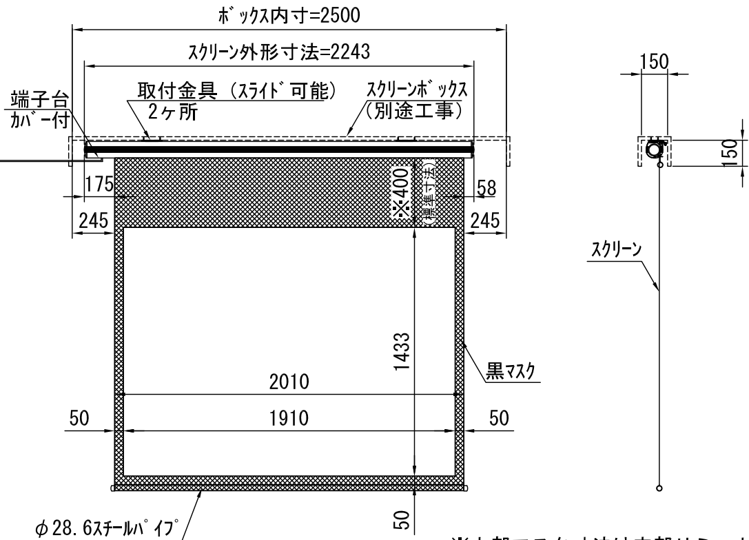
外観図 S=1/30
