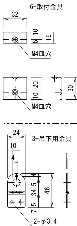
拡大図 S=1/3
