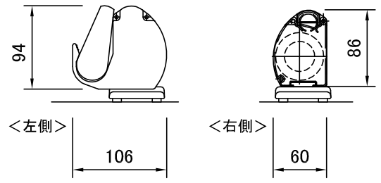
スクリーン収納時ケース外寸 S=1/6
