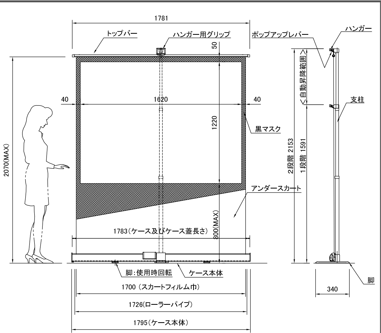
スクリーン設置図 S=1/20
