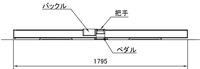
スクリーン収納時ケース外寸 S=1/20
