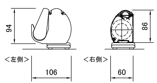
スクリーン収納時ケース外寸 S=1/6
