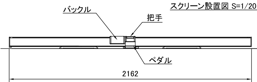
スクリーン収納時ケース外寸 S=1/20
