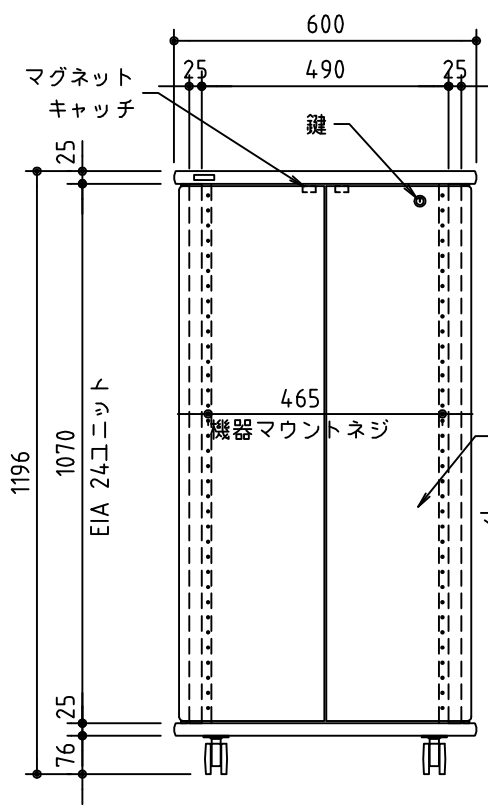
正面
