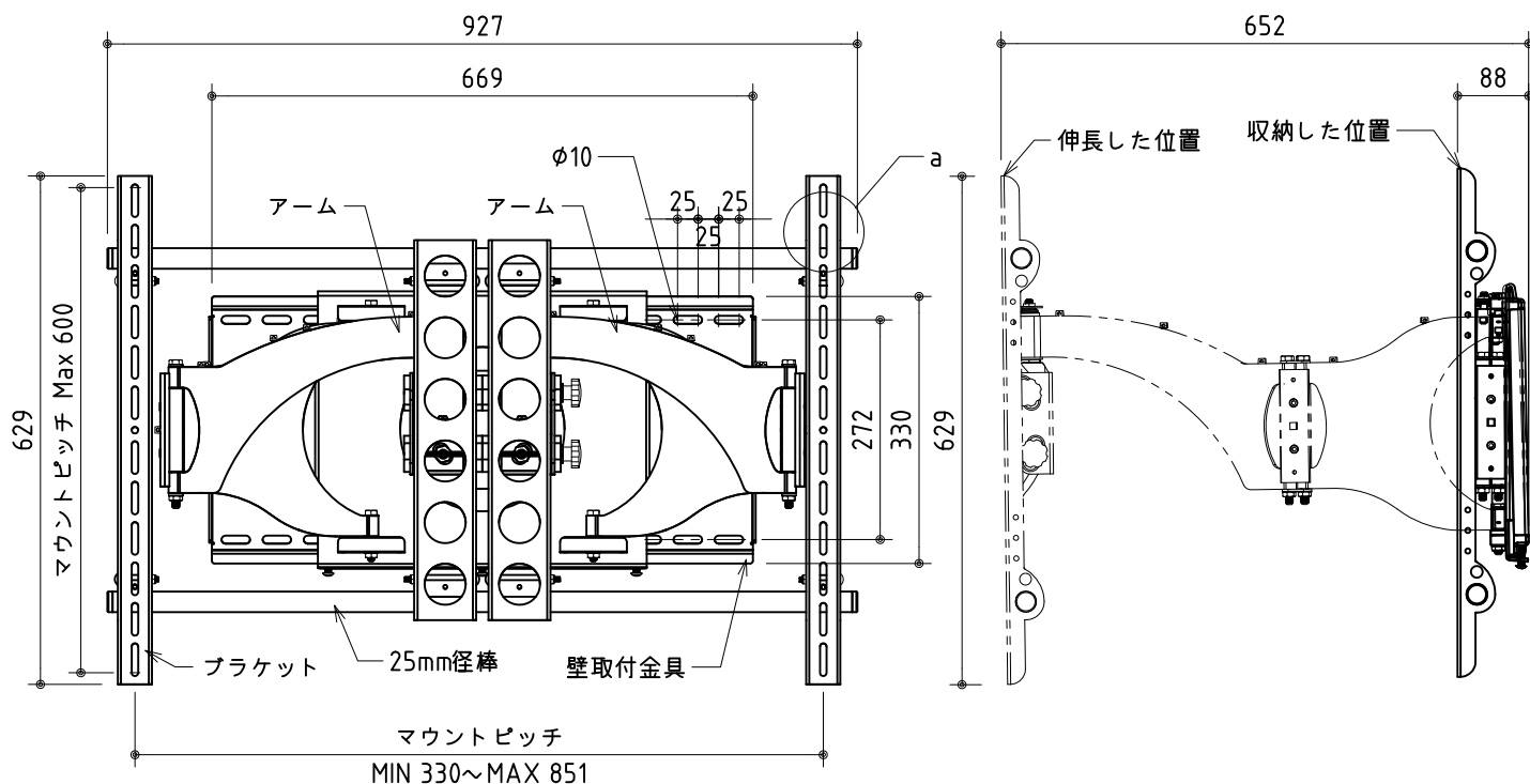
外観図 S = 1/10
