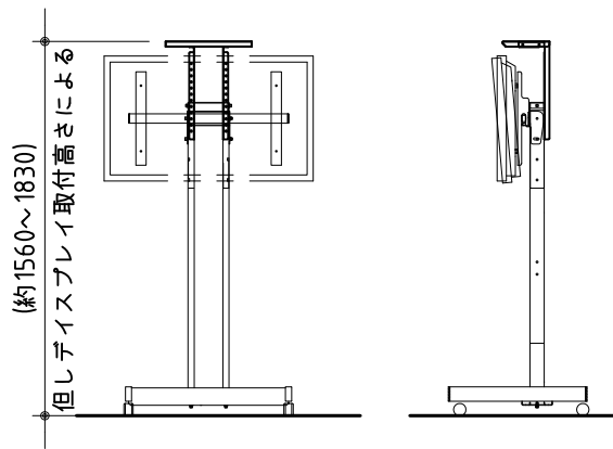
KDS 組込図 1/40
