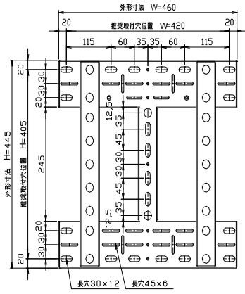
壁面取付ベース金具 (この図面は縮尺ではありません)
